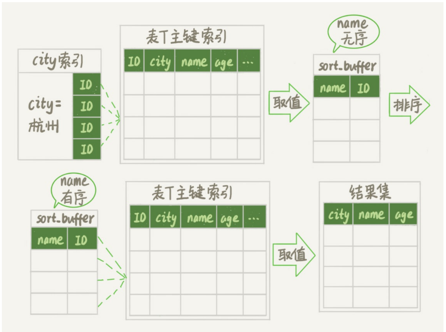
图5 rowid排序
