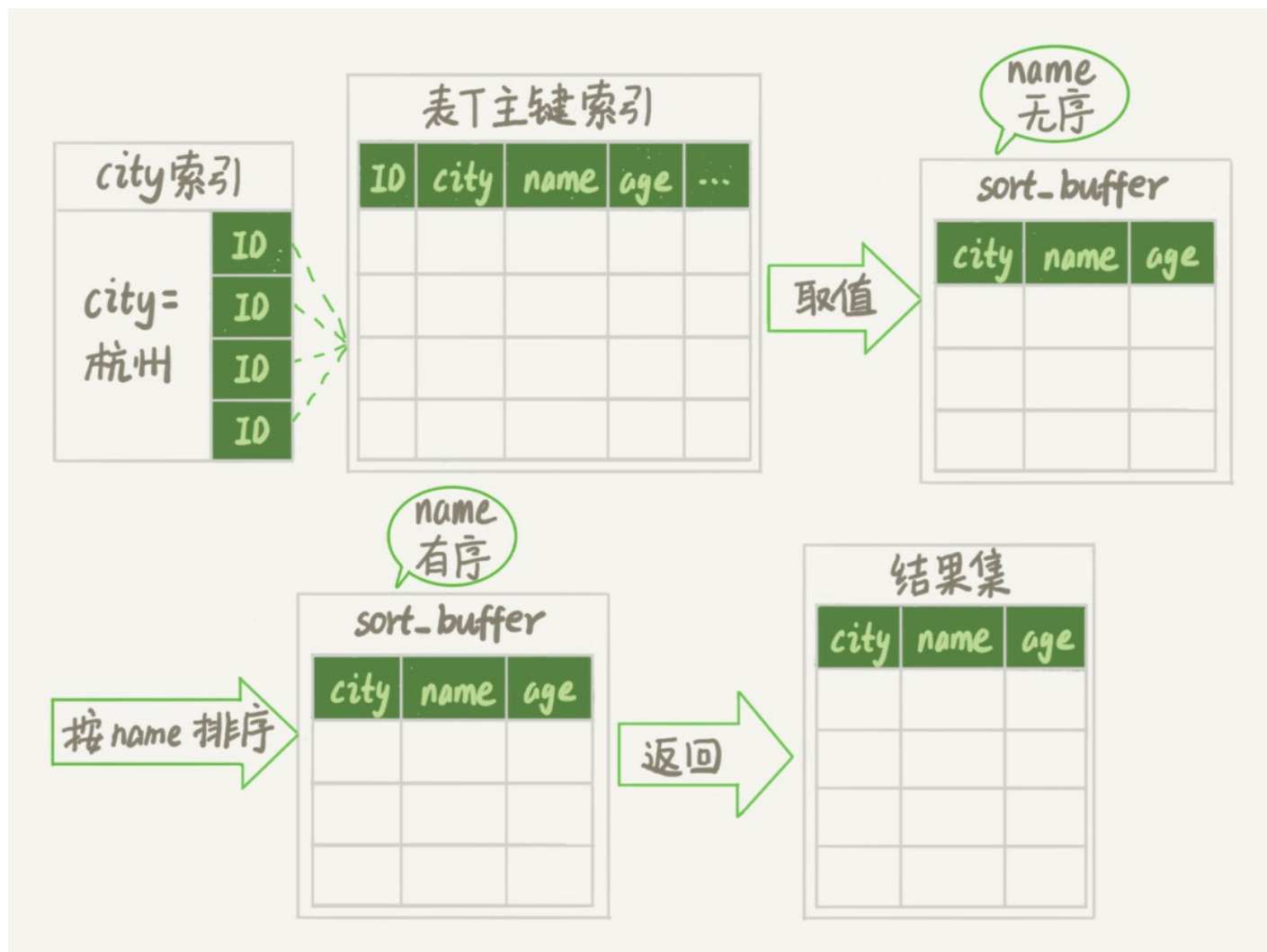
图3 全字段排序
